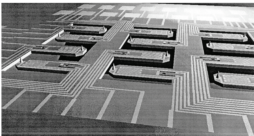
Рис. 9.7. Лабораторная модель многокантилеверной литографической системы для зондового прямого экспонирования
