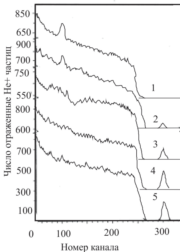
Рис. 3.23. RBS спектры с 1,8 \text{ МэВ He}^+ ПММА, бомбардированном \text{Ag}^+ при дозах ( \text{Ag}^+ ): 0 \text{ мкКл/см}^2 (I); 450 \text{ мкКл/см}^2 (II); 800 \text{ мкКл/см}^2 (III); 2000 \text{ мкКл/см}^2 (IV); 4000 \text{ мкКл/см}^2 (V)
