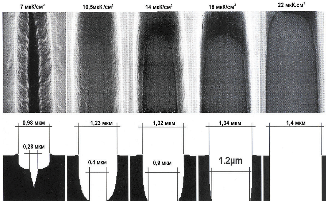
Рис. 8.39. РЕМ микрофотографии – а и соответствующие сечения – б эволюции профилей при различных дозах, если экспонирована 500 нм изолированная линия в 1700 нм (первоначальная толщина резиста) САМР6 (OPD 262)
