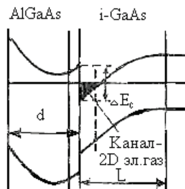
Рис. 1.16. Зонная диаграмма гетероперехода \text{Al}_x\text{Ga}_{1-x}\text{As-GaAs}
