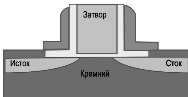
Рис. 1.9. МДП транзистор, выполненный по стандартной технологии
