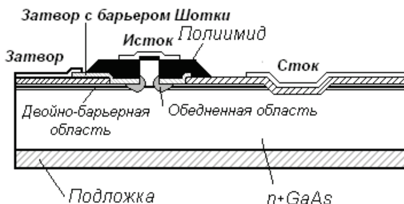
Рис. 2.10. Вертикальный резонансно-туннельный транзистор с кольцевым затвором с барьером Шоттки
