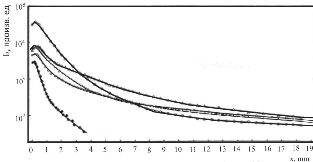
Рис. 3.13. Затухание интенсивности дискретного светового излучения I_d перед бериллиевой мишенью, бомбардированной Ag^+ : 234,8 нм (+); 265,1 нм (●); 313 нм (o); 3321 нм (Δ); 249,5нм (□)
