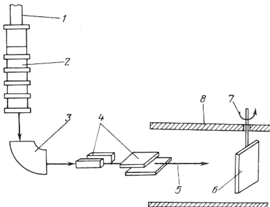
Рис. 6.10. Ионный ускоритель: 1 – вход для ионизируемого вещества; 2 – источник ионов; 3 – магнит для сепарации по Z/M ; 4 – отклоняющая система; 5 – ионный пучок; 6 – образец; 7 – движение приемной кассеты; 8 – приемная камера
