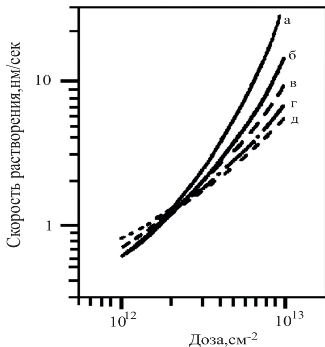
Рис. 8.21. Нелинейная зависимость S(D) для \text{He}^+ , бомбардирующего ПММА. Энергия ионов 80 кэВ. ПММА ( M = 675000 ) проявляется в МИВК/ИПА при 20 °С
