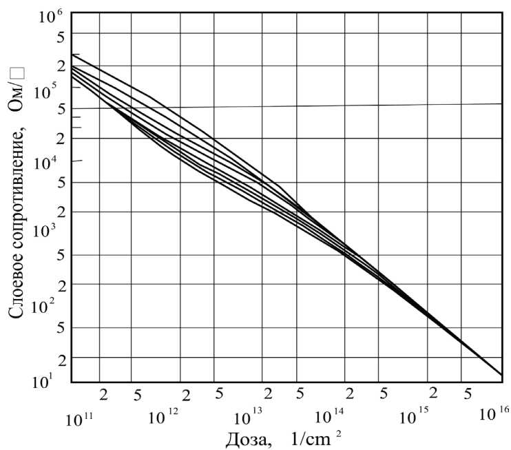
Рис. 6.8. Слоевое сопротивление Si, имплантированным с p -типом примесей. Кривые сверху вниз рассчитаны при допущении нормального распределения, для стандартного отклонения \Delta R_p , мкм: 2,5 \cdot 10^{-3} ; 7,5 \cdot 10^{-3} ; 12,5 \cdot 10^{-3} ; 25 \cdot 10^{-3} ; 75 \cdot 10^{-3} ; 0,1; 0,125; 0,15; 0,175
