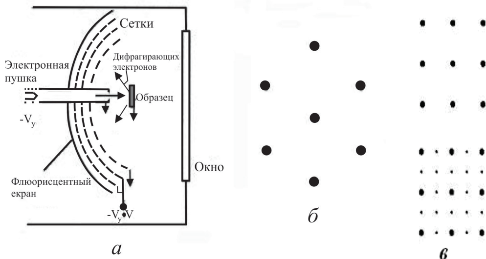
Рис. 3.9. Схема установки для исследования структуры поверхности образцов методом LEED – а; LEED дифракционное изображение при нормальном падении электронов с энергией 80 эВ на Cu (111) – б; LEED дифракционные картины при нормальном падении электронов с энергией 80 эВ на Ni (001): чистого (в –верху) и схемосорбированным кислородом на поверхности (в –внизу)
