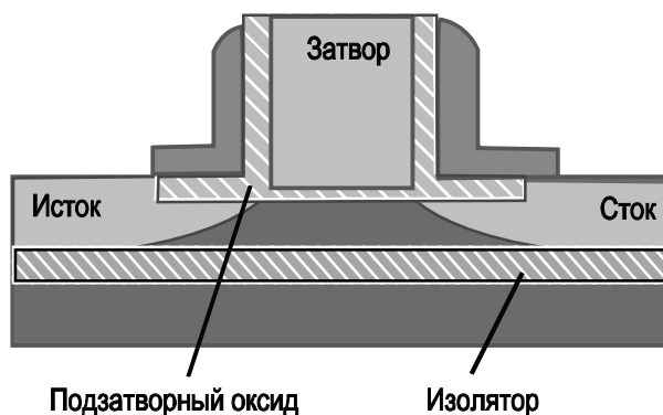
Рис. 1.10. МДП транзистор типа «кремний на изоляторе с сверхтонким телом» (SOI UTBFET)
