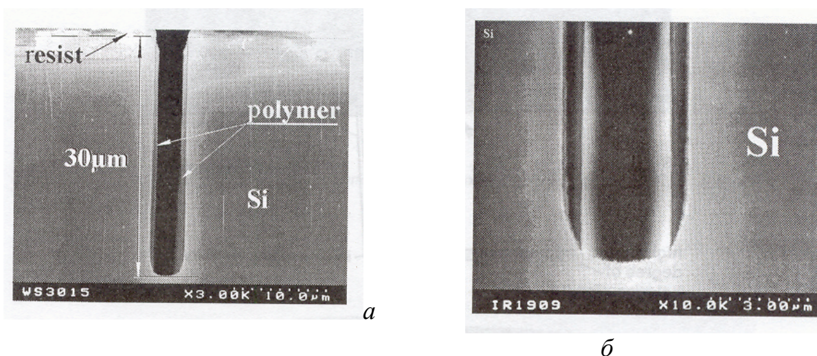
Рис. 5.3. Анизотропное травления Si: а – на стенках отверстия имеется полимер; б – фрагмент анизотропного травления (дно свободное от полимера и стенки с покрытием)
