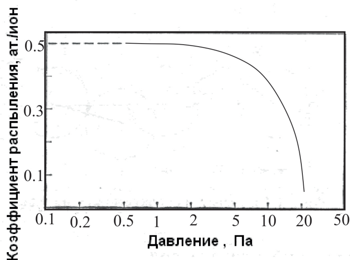
Рис. 4.35. Зависимость коэффициента распыления от давления p газа в камере при бомбардировке мишени из Ni ионами Ag^+ при 150 эВ
