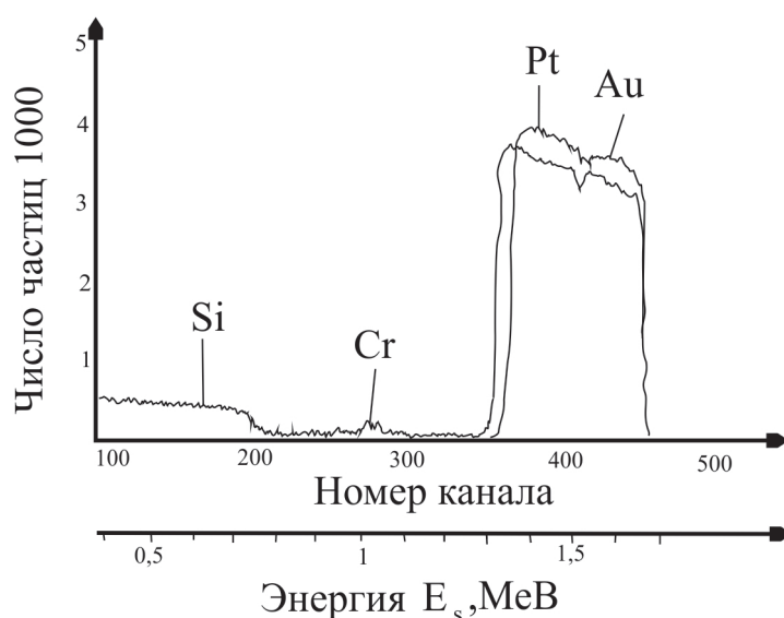
Рис. 3.21. RBS энергетический спектр с 1,8 МэВ \text{He}^+ структуры на рис. 3.15 до и после отжига при 350\text{ }^\circ\text{C}
