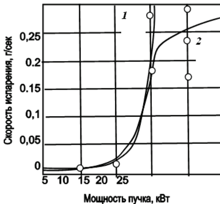
Рис. 4.8. Зависимость скорости испарения от нарастания мощности пучка: 1 – теория, 2 – эксперимент
