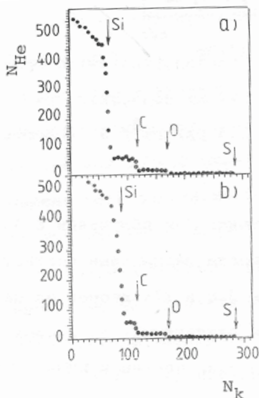
Рис. 3.24. RBS спектры с 1,8 МэВ \text{He}^+ AZ1450 с толщиной 2 мкм в начале анализа – а и после дозы облучения анализирующим пучком 360 \text{ мкКл/см}^2 – б
