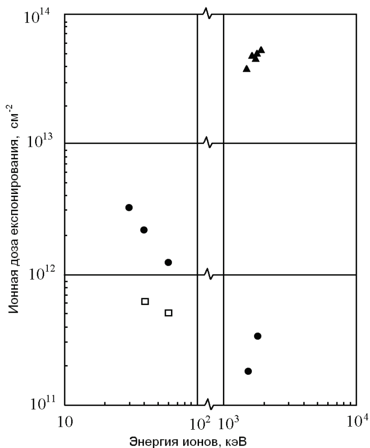
Рис. 8.35. Зависимость чувствительности ПММА от энергии ионов для \text{H}^+ (Δ), \text{He}^+ (●), \text{Ar}^+ (□)
