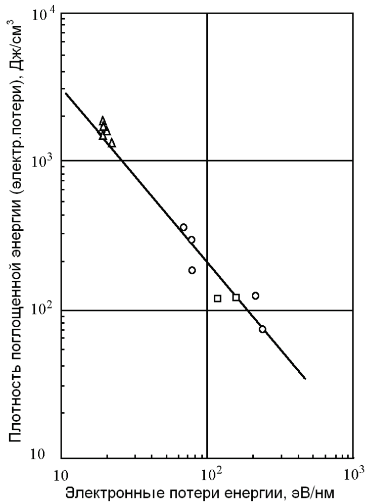
Рис. 8.36. Абсорбированные (dE/dx)_{э1} для единицы объема при D_0 от (dE/dx)_{э1} для использованных ионов H^+(\Delta) , He^+(\bullet) , Ag^+(\square)
