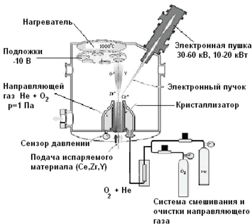
Рис. 4.10. Принципиальная схема ассистированного плазмой направленного нанесения пленок из паровой фазы
