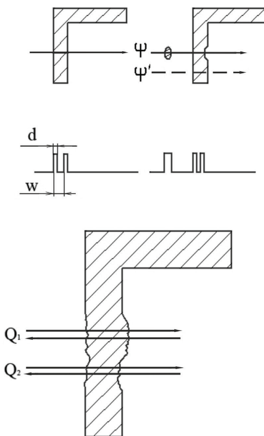
Рис. 8.8. Принципиальная схема распознавания сигналов с реперов
