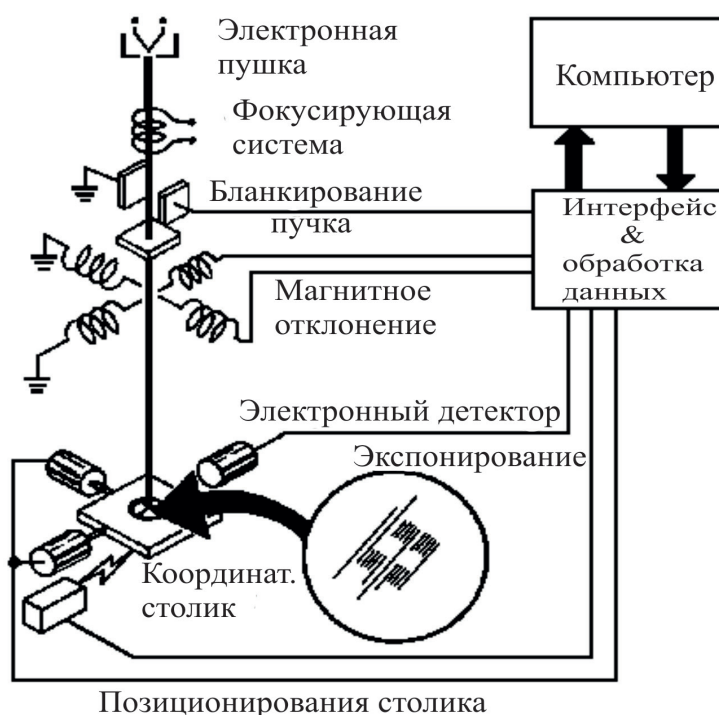
Рис. 8.2. Блок-схема литографической системы с директным последовательным экспонированием гауссовым пучком
