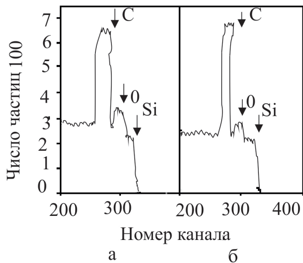
Рис. 3.22. RBS спектр с 1,5 \text{ МэВ H}^+ от ПММА, с толщиной 2 \text{ мкм} в начале – а и после дозы 1020 \text{ мкКл/см}^2 – б
