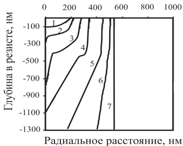
Рис. 8.37. Смоделированные профили проявленного резиста для одной 0,5 мкм изолированной линии в резисте толщиной 0,5 мкм, нанесенные на пленки из 0,08 мкм Cr, отложенного на толстом слое SiO 2 . Экспонирующий луч является гауссовым с дисперсией \sigma = 50 нм
