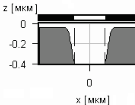
Рис. 8.46. Максимальный угол наклона боковых стенок 63,6^\circ при применении оптимизационного критерия I
