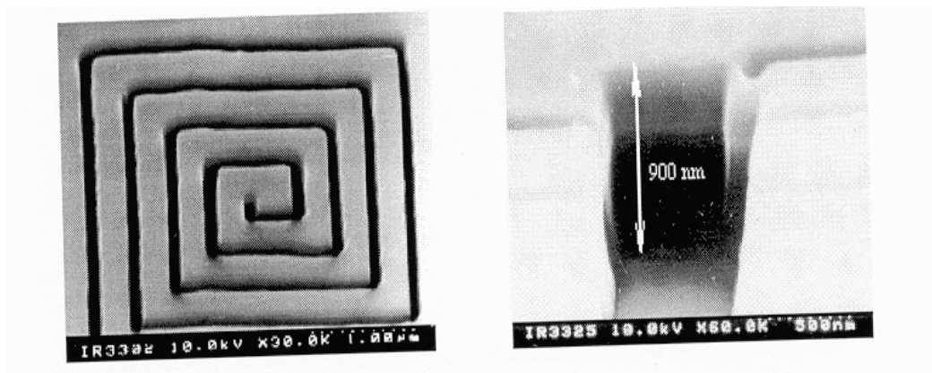
Рис. 9.6. Рисунок с линией шириной 60 нм, изготовленный STM. Травление в кремниевой пластине, покрытой с Al/a-C:H. Глубина травления 900 нм, что соответствует отношению глубины к ширине линии (aspect ratio), превышающему 10
