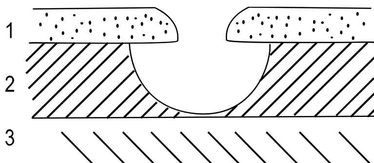
Рис. 5.1. Типичный профиль химического травления: 1 – резист; 2 – вытравливаемый слой; 3 – подложка
