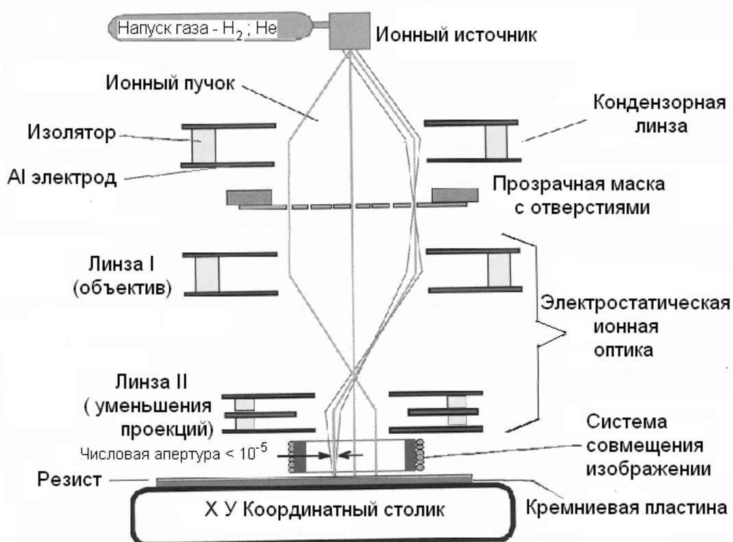
Рис. 8.14. Принципиальная схема проекционной системы для ионной литографии
