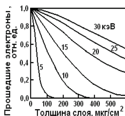
Рис. 7.9. Кривые ослабления электронного тока (5–30 кэВ) прошедших электронов, бомбардирующих тонкие пленки меди в зависимости от их толщины
