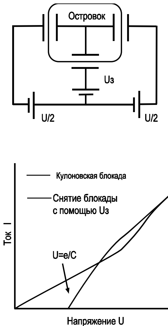
Рис. 2.13. Одноэлектронный полевой транзистор с двумя симметричными туннельными переходами. На затвор подается напряжение U_3 . Внизу рисунка – вольт-амперные характеристики прибора
