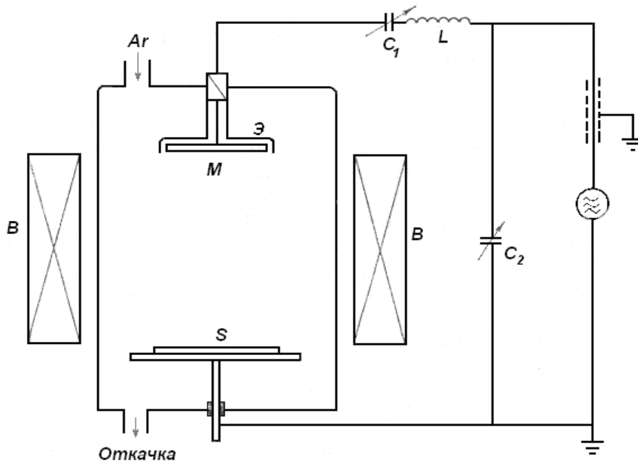
Рис. 4.38. Принципиальная схема установки диодного типа для ВЧ-распыления: M – мишень; \mathcal{E} – экранирующий электрод; S – подложка; L и C_1 – согласующее устройство
