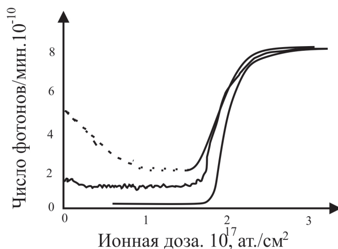
Рис. 3.17. Интенсивность линии Si атомов до отжига (внизу), после отжига при 350 °С, 10 мин (середина) и при 400 °С, 10 мин (верх), структуры, исследуемой на рис. 3.15
