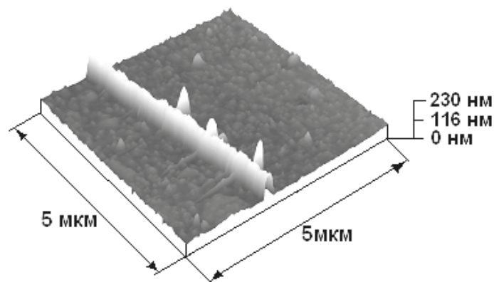
Рис. 8.42. AFM микрофотография линии (шириной 500 нм), проявленной в резисте. Подложка из \text{YBa}_2\text{Cu}_3\text{O}_7 ; экспонирование электронами с энергией 30 кэВ
