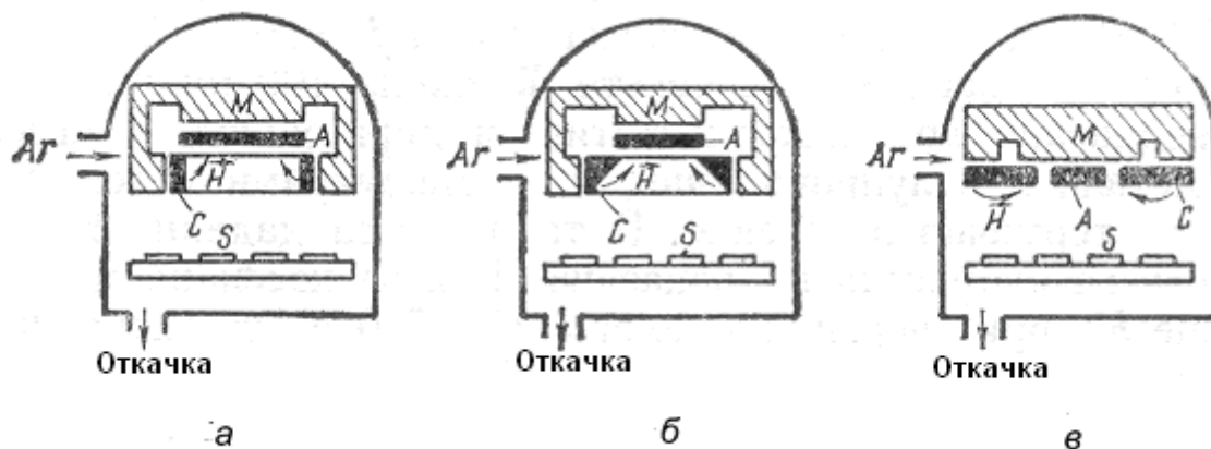
Рис. 4.39. Типичные конструкции магнетронов для распыления: a – цилиндрическая; b – коническая конструкции катодов; v – планарный катод; C – катод; S – подложка; A – анод
