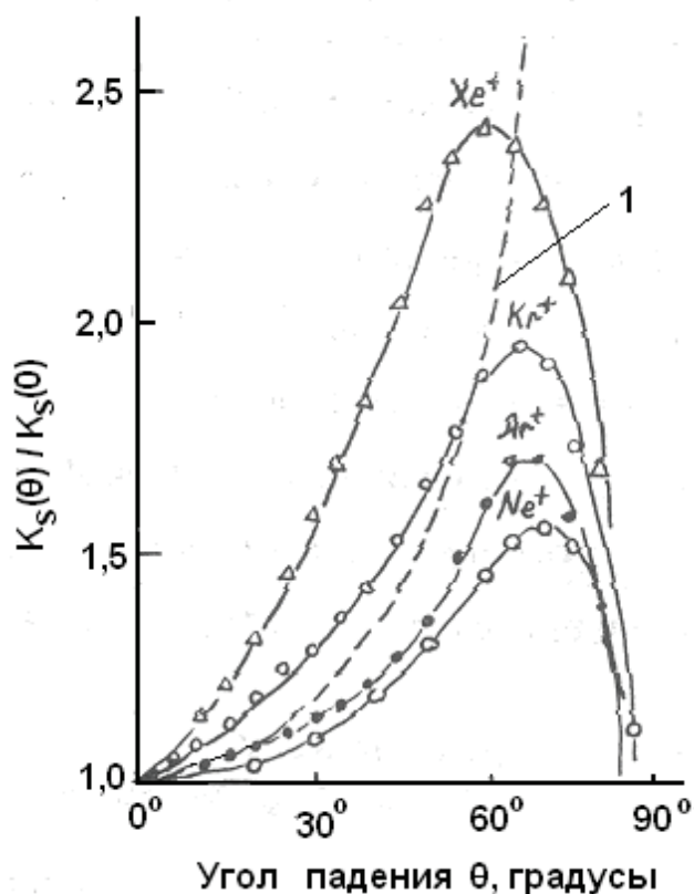
Рис.4.34. Зависимость коэффициента распыления разными ионами от угла падения \theta : мишень из Cu, E = 1,05 кэВ; кривая 1 – K_S(\theta)/K_S(0) \sim (\cos)^{-1}
