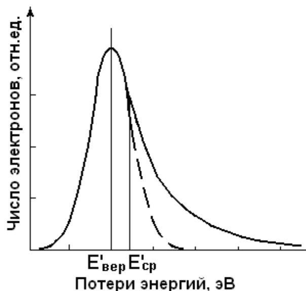
Рис. 7.7. Распределение потери энергии электронов, прошедших через слой x , E'_{\text{ср}} – средняя потеря энергии, E'_{\text{вер}} – энергия вероятных потерь
